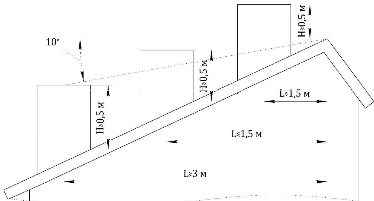
Рисунок 11 - Варианты расположения трубы на скате
